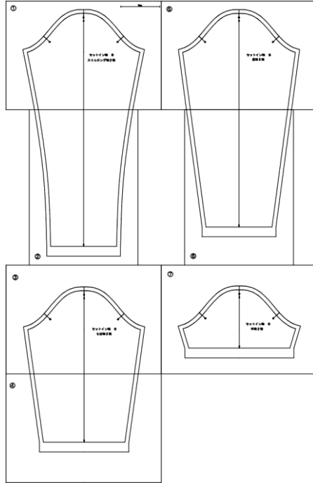
袖(A3判 7枚)
